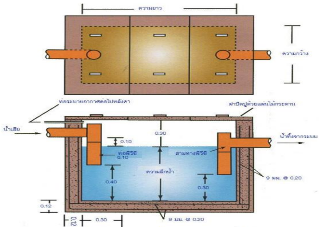
บ่อดักไขมันแบบสร้างในที่สำหรับอาคารขนาดใหญ่
