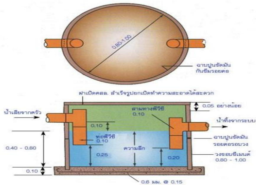
บ่อดักไขมันแบบวงขอบซีเมนต์สำหรับบ้านพักอาศัย
