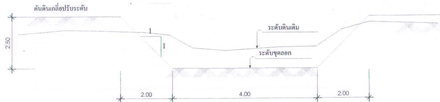
รูปตัดตามขวาง แสดงสัดส่วนการขุดลอก STA 2+000 - STA 3+000
