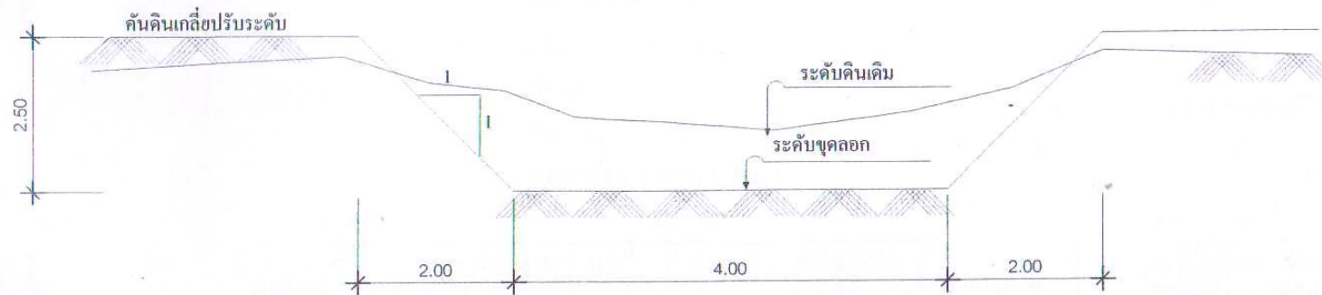
รูปตัดตามขวาง แสดงสัดส่วนการขุดลอก STA 1+000 - STA 2+000
