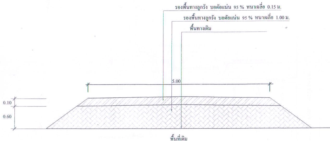
รูปตัดถนนลูกรัง (ก) - (ก) มาตราส่วน 1:50
